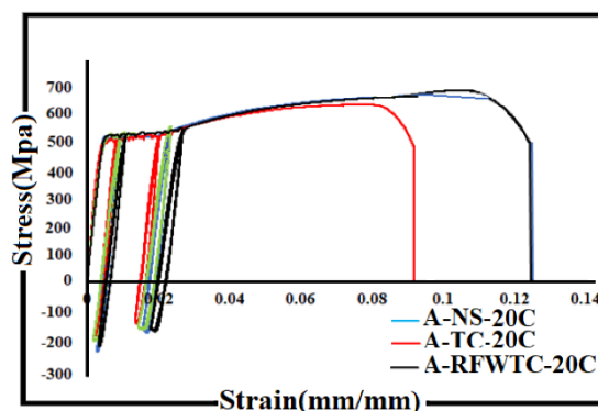
شکل ۴: نمودار \sigma - \epsilon نمونه‌های بدون غلاف بتنی (NS, TC, RFWTC) تحت بارگذاری چرخه‌ای
