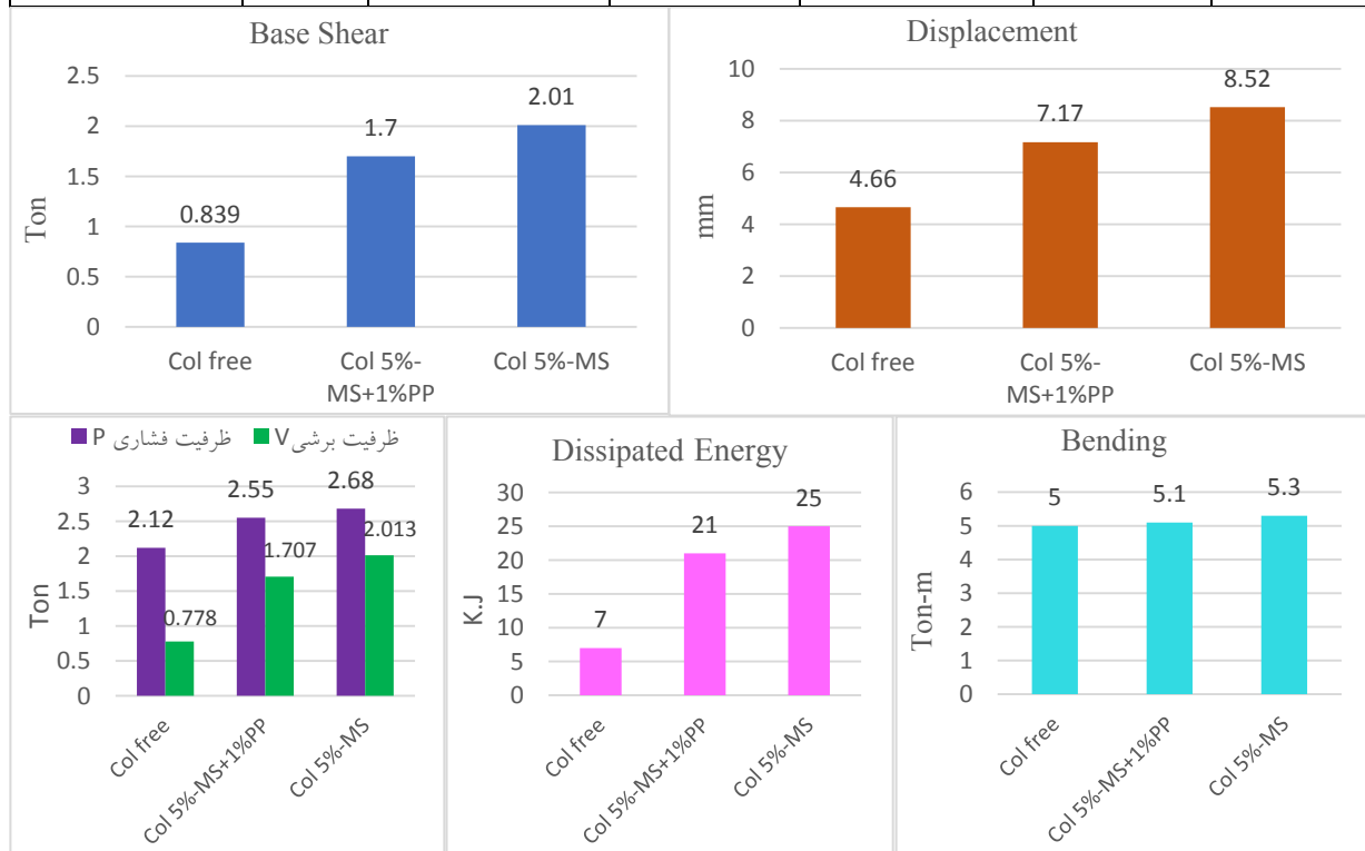
شکل (۵) - نمودار نتایج مربوط به ستونهای ساخته شده تحت اثر رکورد زلزله Northridge ایستگاه Sylmar
