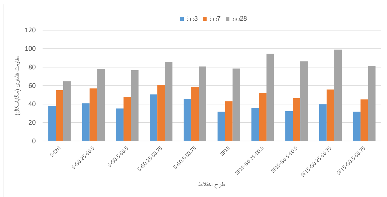
شکل ۳- مقاومت فشاری نمونه ها مختلف در سنین ۳، ۷ و ۲۸ روز
